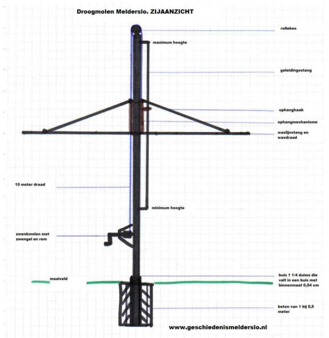
Schematische tekening van de Melderse Droogmolen.
