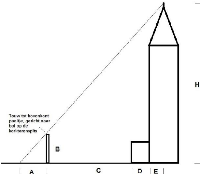
Schematisch overzicht meting kerk Melderslo.
